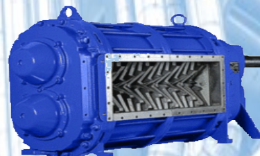
X Ripper
